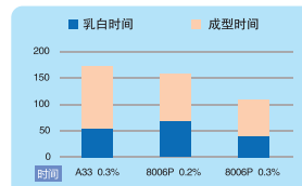
图1-8 催化剂对泡沫成型时间的影响对比
