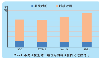
图2-1 不同催化剂对三组份筛网料催化固化过程对比
