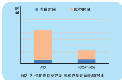
图2-2 催化剂对材料乳白和成型时间影响对比
