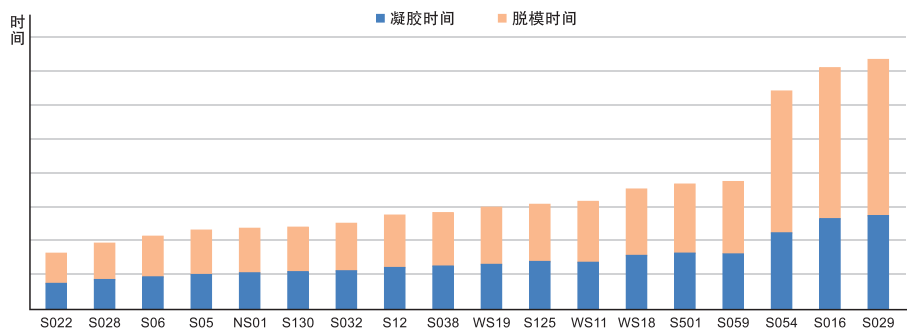
图1-2 TCAT系列特种有机锡催化活性对比 (测试体系: PAPI+PPG)
